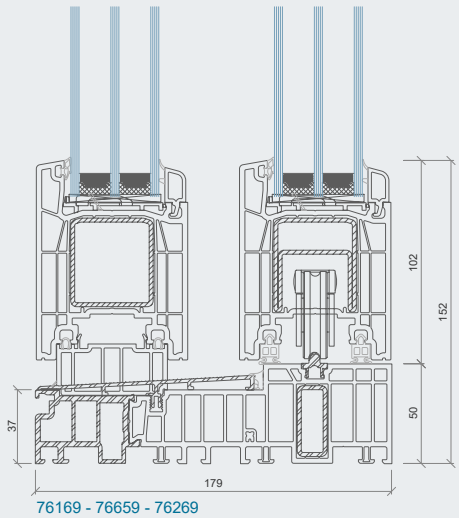
Sección PremiDoor76
